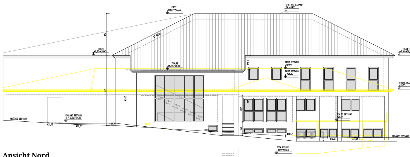
Ansicht Nord
