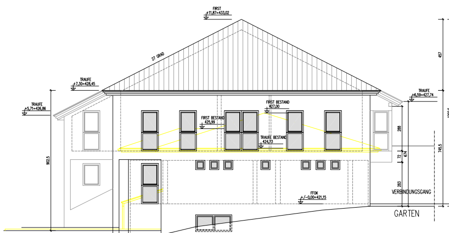
Ansicht West
